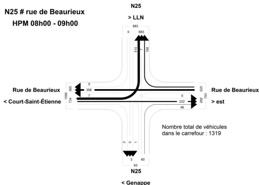
Figure 287 : Diagramme des flux (en evp) au carrefour situé N25 # rue de Beaurieux (est) à l'heure de pointe du matin, entre 08h00 et 09h00
