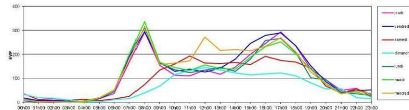
Figure 240. Comptages de circulation Poste 041
