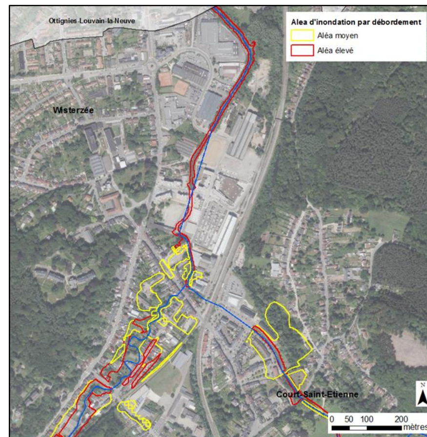
Figure 59: Aléa d'inondation par débordement moyen et élevé à l'ouest de Court-Saint-Etienne (Source : SPW, 2016)
