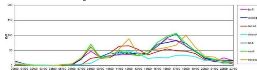
Figure 252. Comptages de circulation Poste 071
