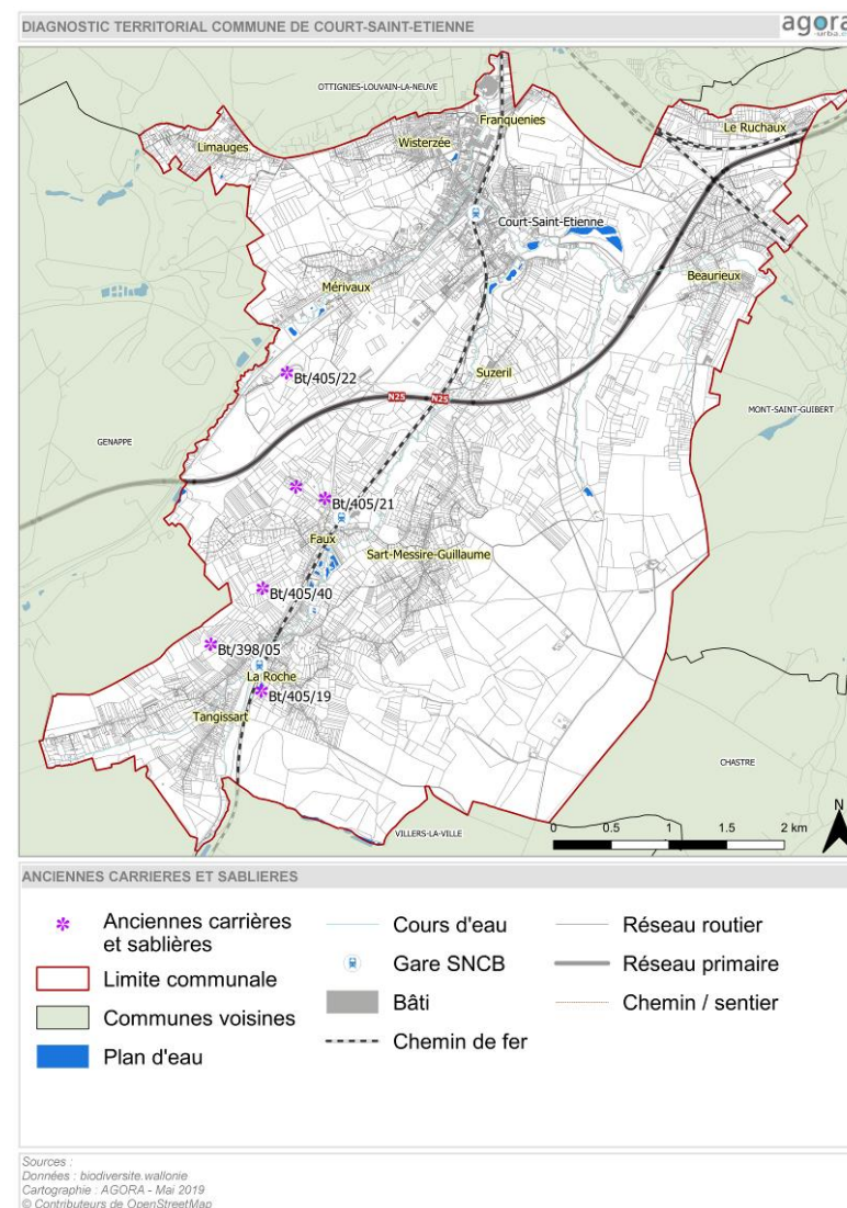
Figure 41 : Localisation des anciennes sablières et carrières (Source : SPW ; cartographie : AGORA)
