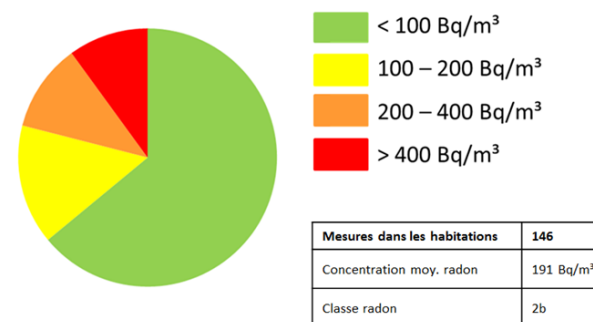
Figure 40 : Graphique de la répartition des concentrations en radon mesurées à l'intérieur des maisons (Source : AFCN – Agence Fédérale de Contrôle Nucléaire)
