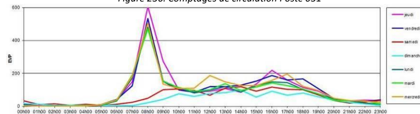
Figure 237. Comptages de circulation Poste 032
