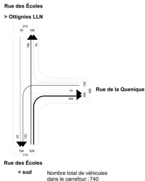
Figure 281 : Diagramme des flux (en evp) au carrefour situé rue des Écoles # rue de la Quenique à l'heure de pointe du matin, entre 08h00 et 09h00
