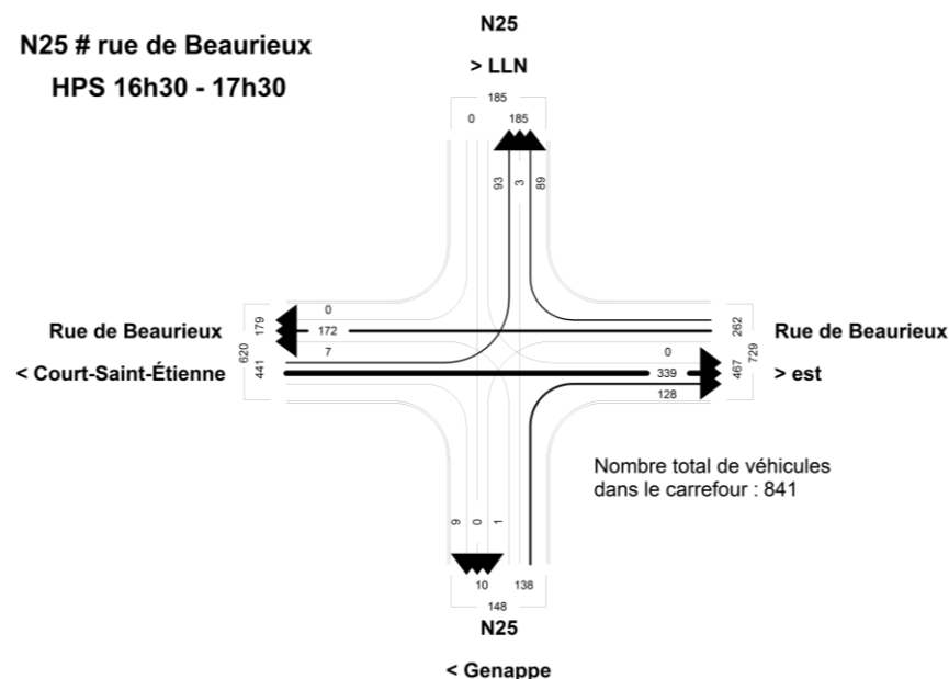
Figure 288 : Diagramme des flux (en evp) au carrefour situé N25 # rue de Beaurieux (est) à l'heure de pointe du soir, entre 16h30 et 17h30
