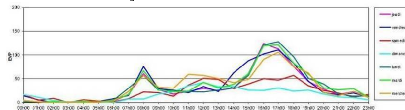
Figure 260. Comptages de circulation Poste 091
