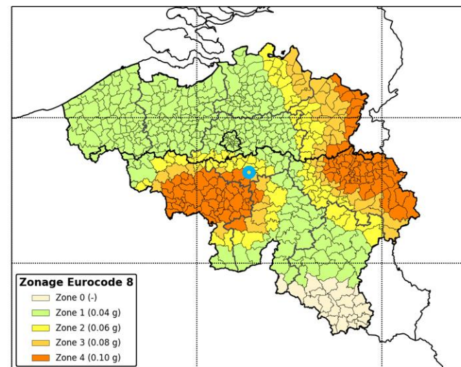
Figure 38 : Carte du zonage du territoire belge pour l'Eurocode 8 issue de l'Annexe Nationale Belge (Source : Observatoire Royal de Belgique)
