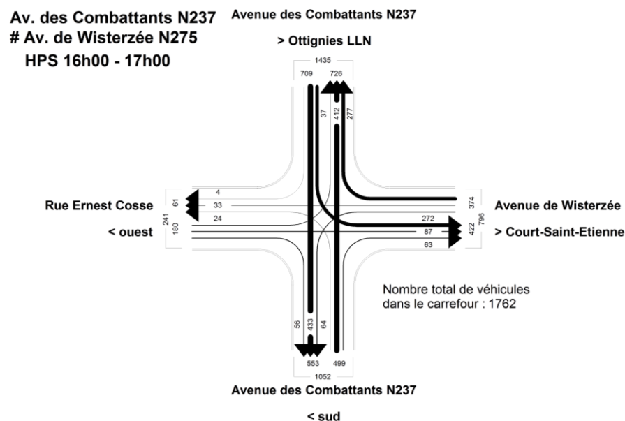
Figure 272 : Diagramme des flux (en evp) au carrefour situé N237 # N275 à l'heure de pointe du soir, entre 16h00 et 17h00
