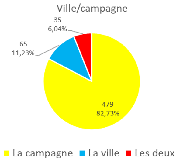
Figure 217: Répartition ville/campagne
