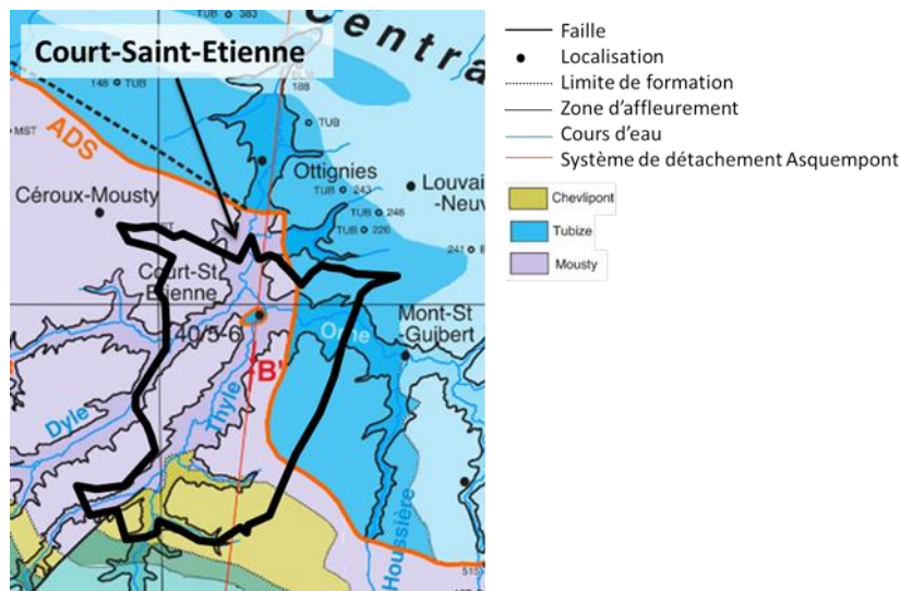
Figure 37 : Localisation géologique de la commune de Court-Saint-Etienne (Source : A. Herbosch & T. Debacker, 2018)
