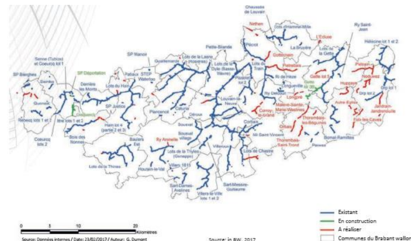
Figure 403: Les collecteurs du réseau d'assainissement d'in BW en Brabant wallon
