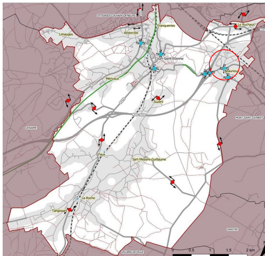
Figure 278. Comptages directionnels rue de Beaurieux – rue de la Papeterie
